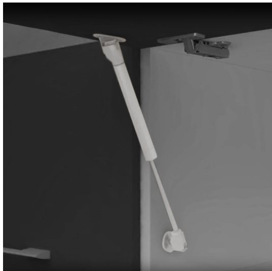
Emuca Pistone a gas per ante a ribalta verso l'alto, forza 5 kg, corsa 80 mm, Grigio
